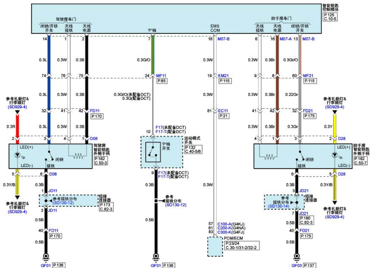
智能钥匙模块系统(4)
